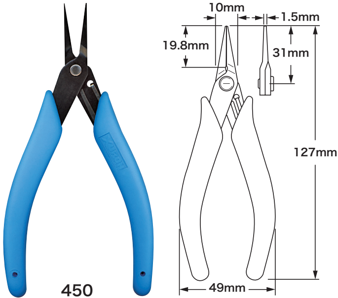
450型 ピンセットタイプ・プライヤ
