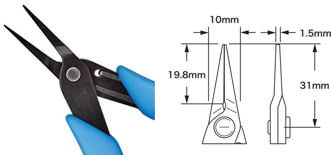
450型 ピンセットタイプ・プライヤ
