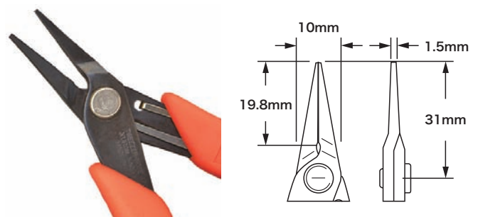
450S型 ギザ付ピンセットタイプ・プライヤ
