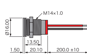
ショートボディワイヤ
