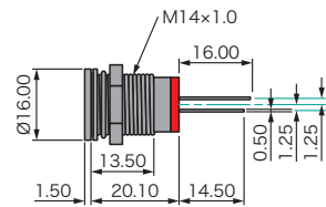
ショートボディリード
