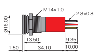
ハンダラグ/ファストン
