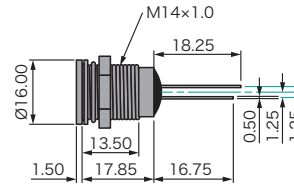
背面エポキシ封止リード
