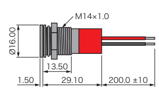
ワイヤ
