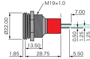
背面エポキシ封止リード
