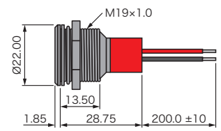
背面エポキシ封止ワイヤ
